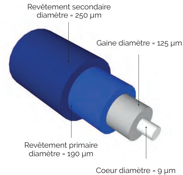
Fig. 116 | Structure d'une fibre optique (Rappel : 1 \mu\text{m} = 0,001 \text{ m m} )
