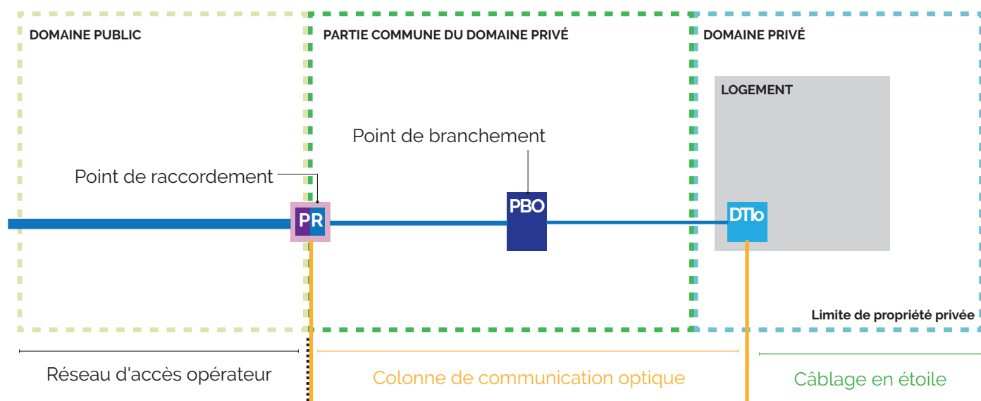
Fig. 114 | Synoptique d'une colonne de communication
