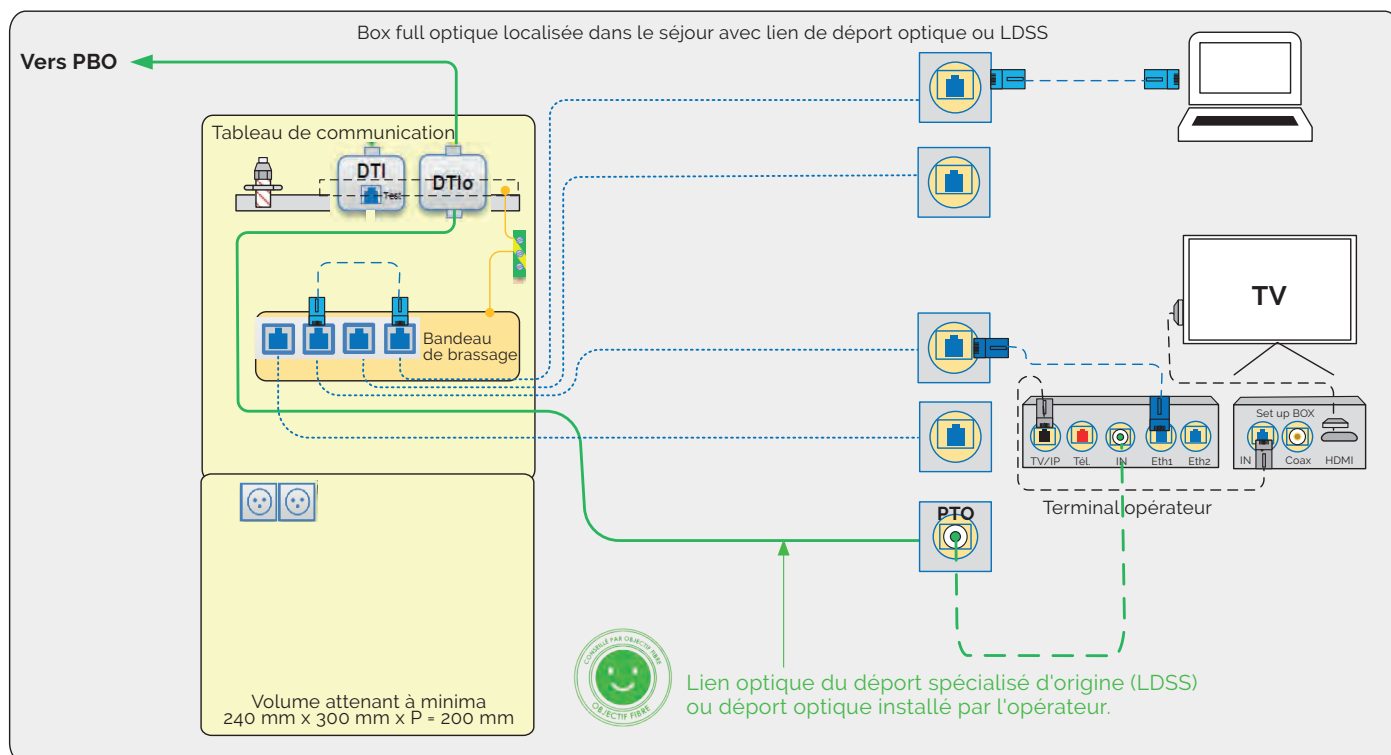
Fig. 75 | Distribution du logement avec une box full optique localisée dans le séjour et lien de déport optique
