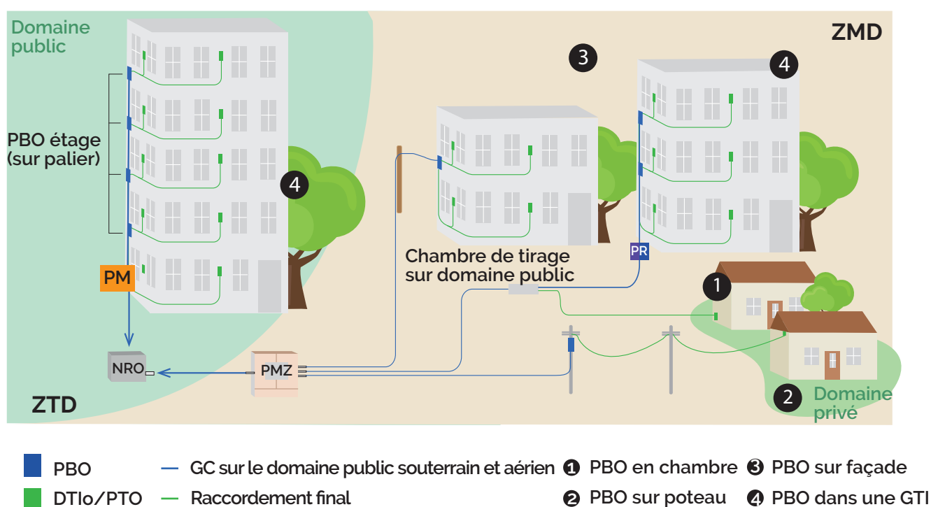
Fig. 07 | Synthétique du déploiement de la boucle locale optique mutualisée (ZTD et hors ZTD)
