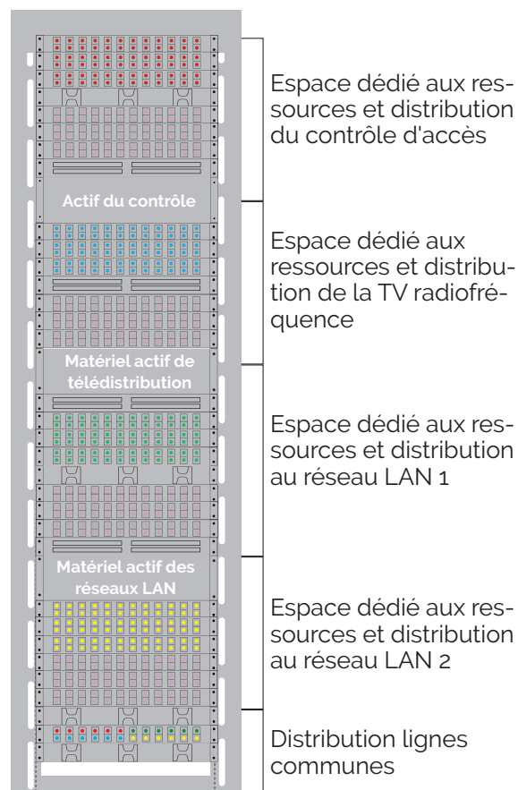
Fig. 101 | Exemple de composition d'un point de raccordement optique de services
