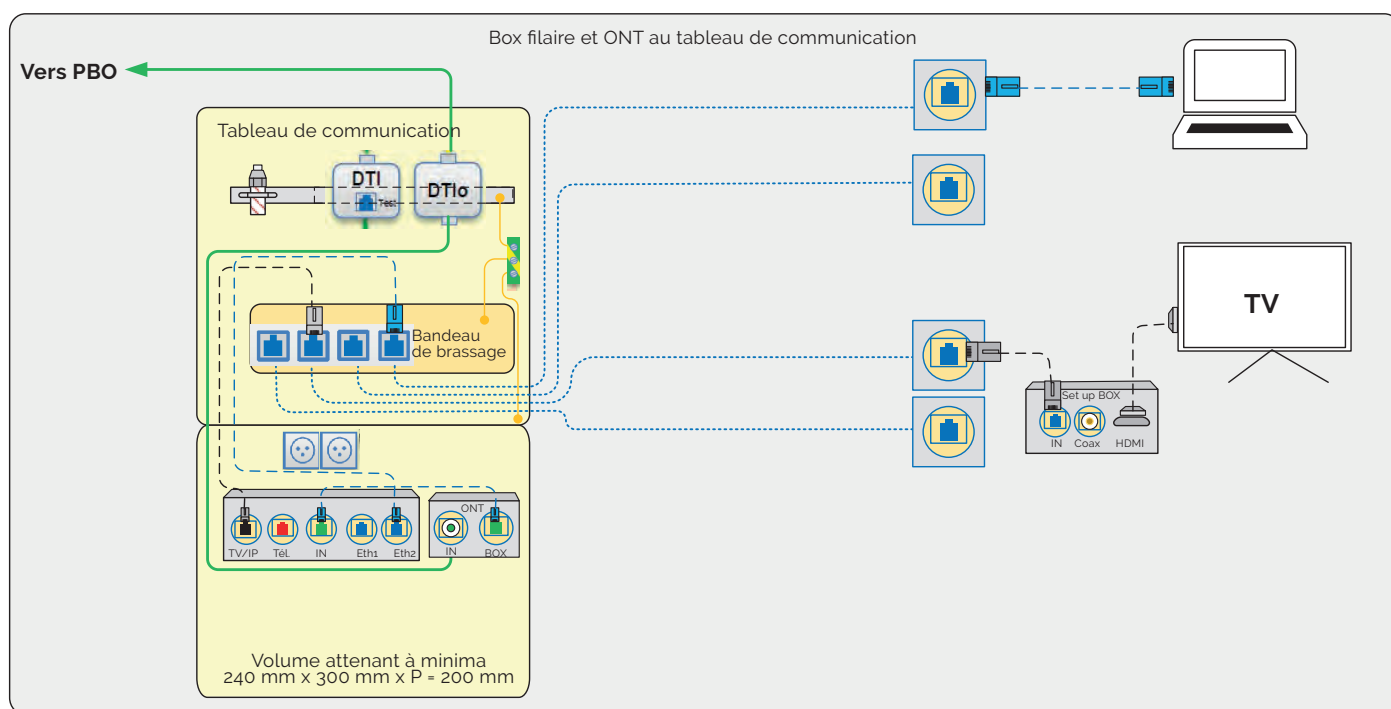
Fig. 73 | Distribution du logement avec une box avec ONT séparées au TC
