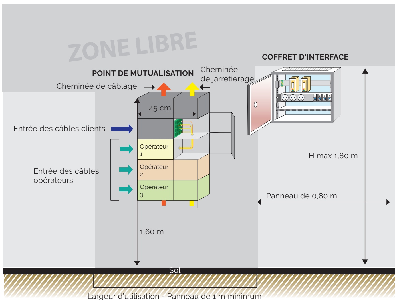
Fig. 27 | Exemple d'implantation de matériels dans un local technique d'un immeuble de ZTD
