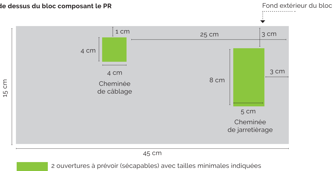
Fig. 138 | Vue de dessus du bloc pour coffret de mutualisation catégorie C, situé en immeuble
