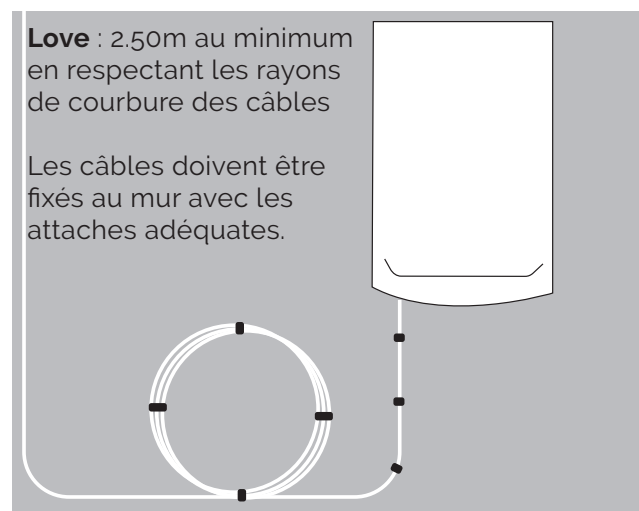
Fig. 42 | Exemple de lovage de câble de la colonne de communication en sortie d'un PR
