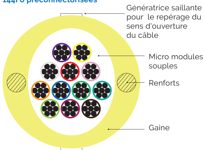
Fig. 143 | La capacité en fibres peut aller jusqu'à 144Fo préconnectorisées
