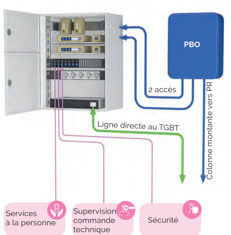
Fig. 66 | Synoptique des différents branchements du coffret de services
