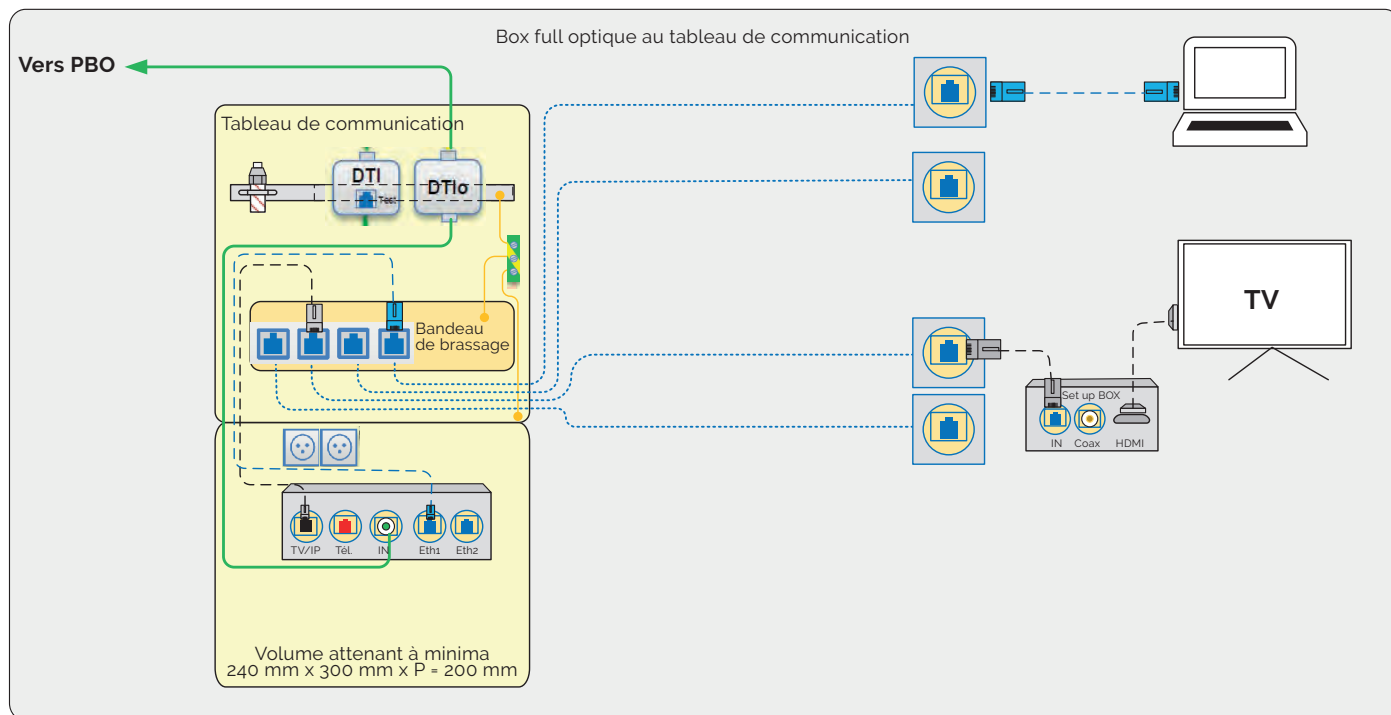
Fig. 72 | Distribution du logement avec la box full optique centralisée au tableau de communication
