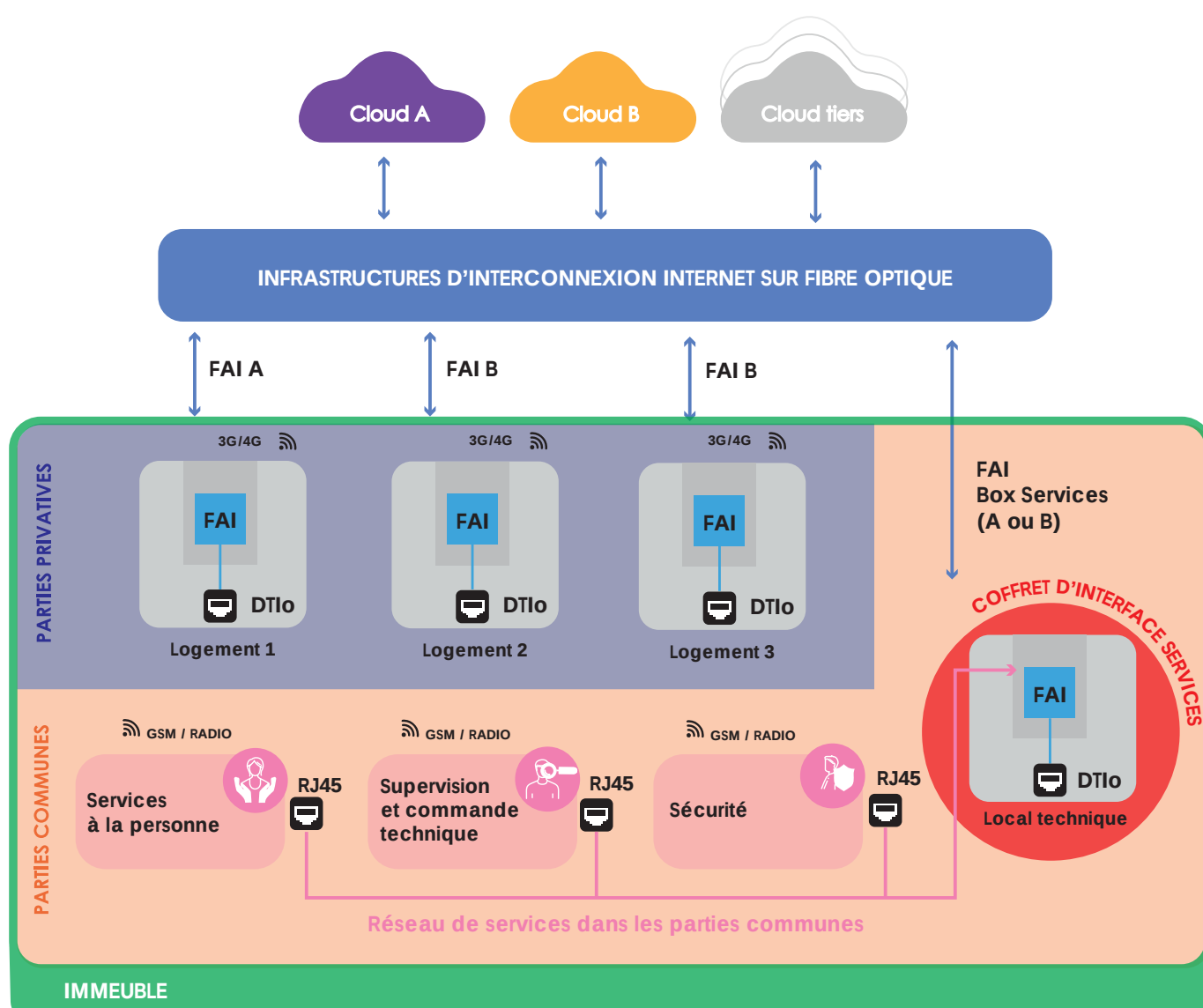
Fig. 83 | Organisation générale des services de l'immeuble
