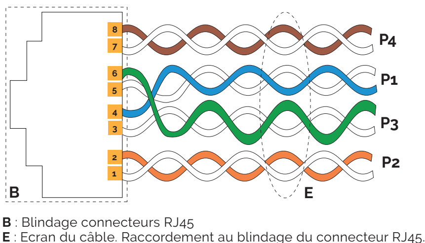
Fig. 70 | Principe de raccordement des socles de prises RJ45
