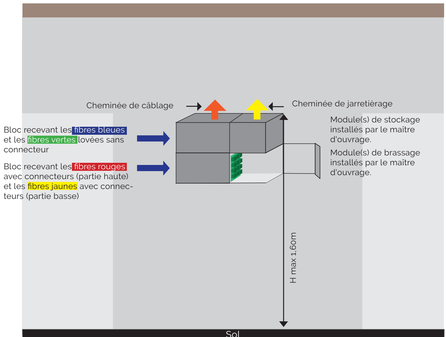
Fig. 58 | Exemple de rangement de câbles dans un PR constitué de blocs
