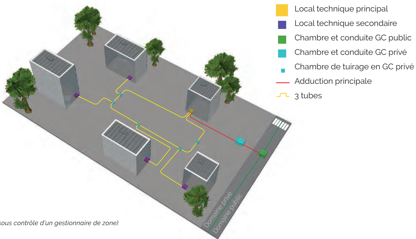
Fig. 20 | Adductions d'un campus privé 1 suivant le principe d'une structure en boucle
