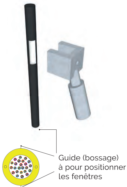
Fig. 139 | Ouverture de fenêtres dans les câbles de la colonne montante
