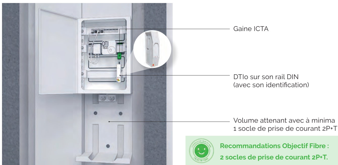
Fig. 37 | Arrivée du kit DTIo et son installation dans le TC
