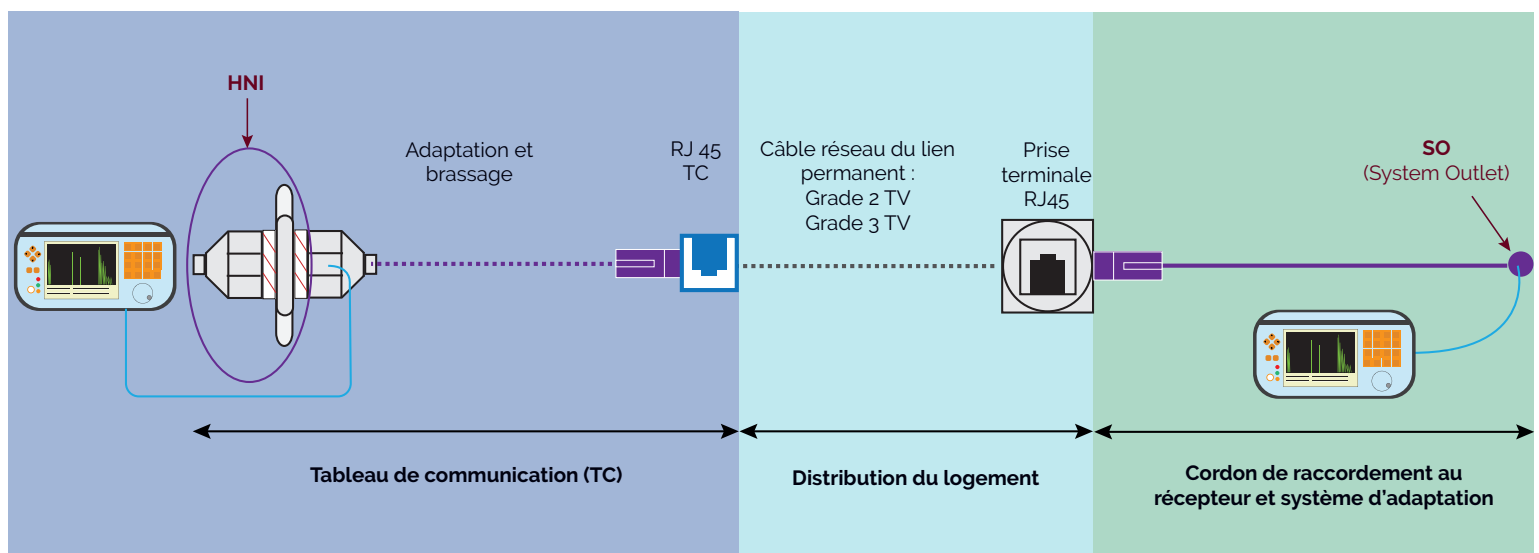
Fig. 113 | Le test du câblage résidentiel
