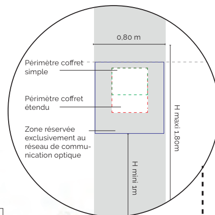
Fig. 87 | Implantation d'un coffret de communication étendu dans le local d'un campus
